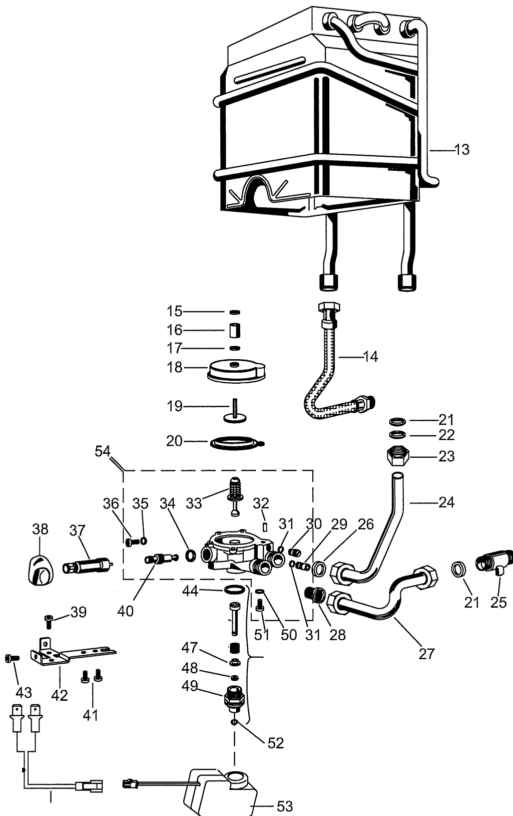
CIRCUITO ACQUA
