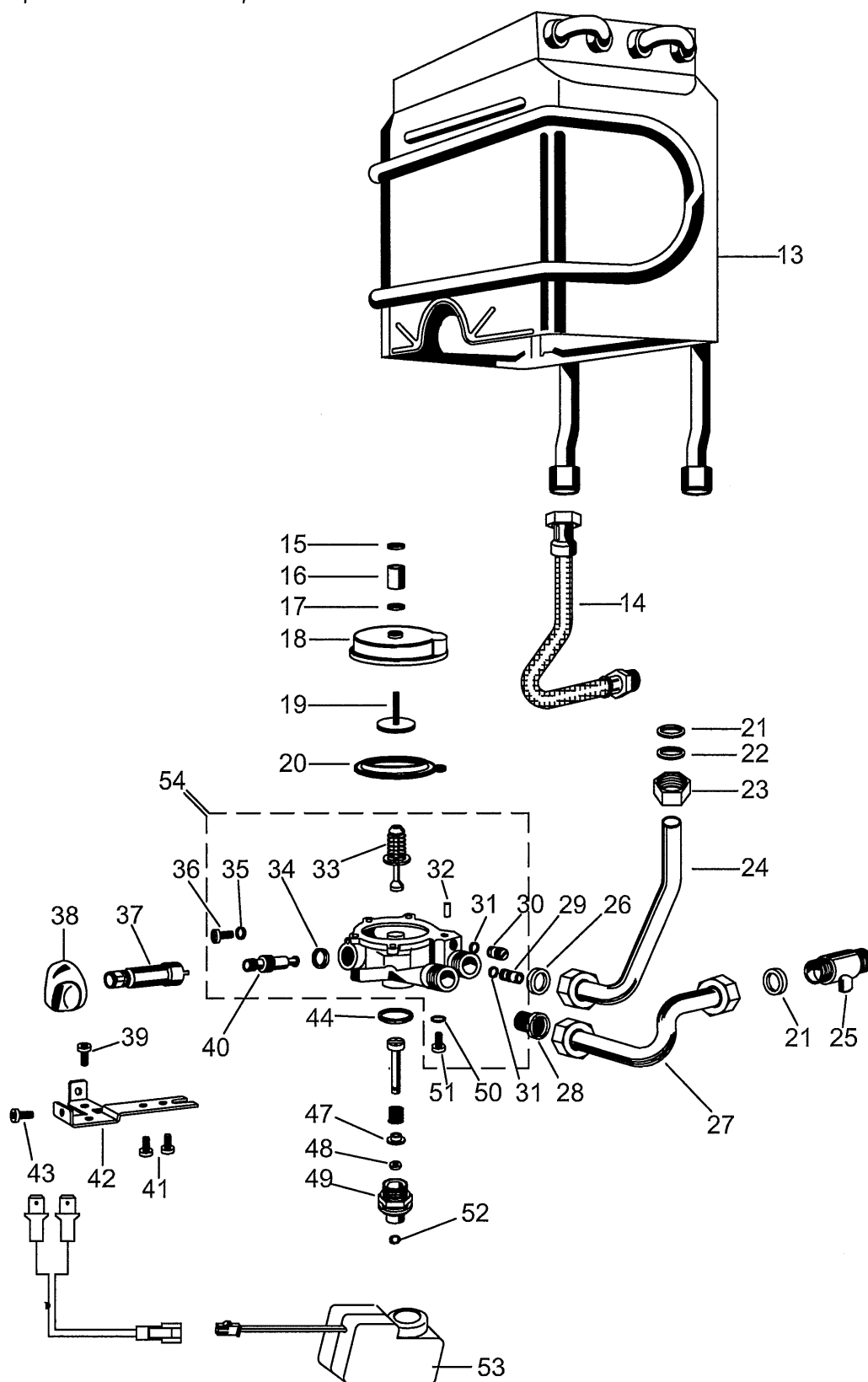
CIRCUITO ACQUA
